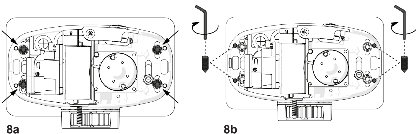
Fig. 8 IT - Fissaggio della piastra EN - Installing the foundation box FR - Fixation de la plaque de fondation ES - Instalación de la caja de cimentación
