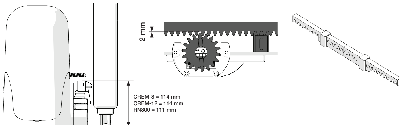
Fig. 10 IT - Fissaggio cremagliera EN - Rack assembling FR - Pose de la crémaillère ES - Fijación de la cremallera
