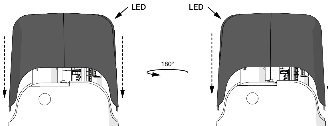
Fig. 9 IT - Chiusura del coperchio EN - Closing the cover FR - Fermeture du couvercle ES - Cierre de la tapa
